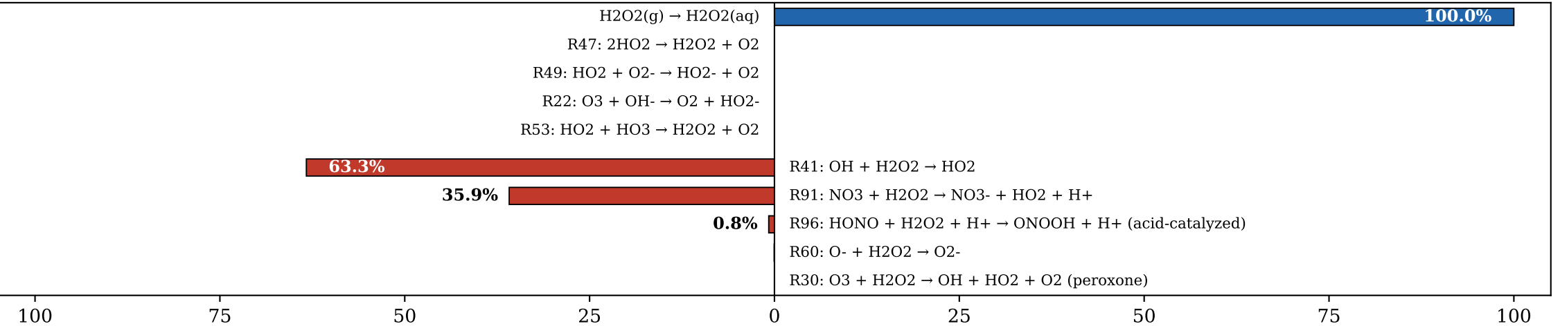
(d) \text{H}_2\text{O}_2 ( \Sigma\text{src} = 7.33\text{e-}08 \text{ M/s} )
